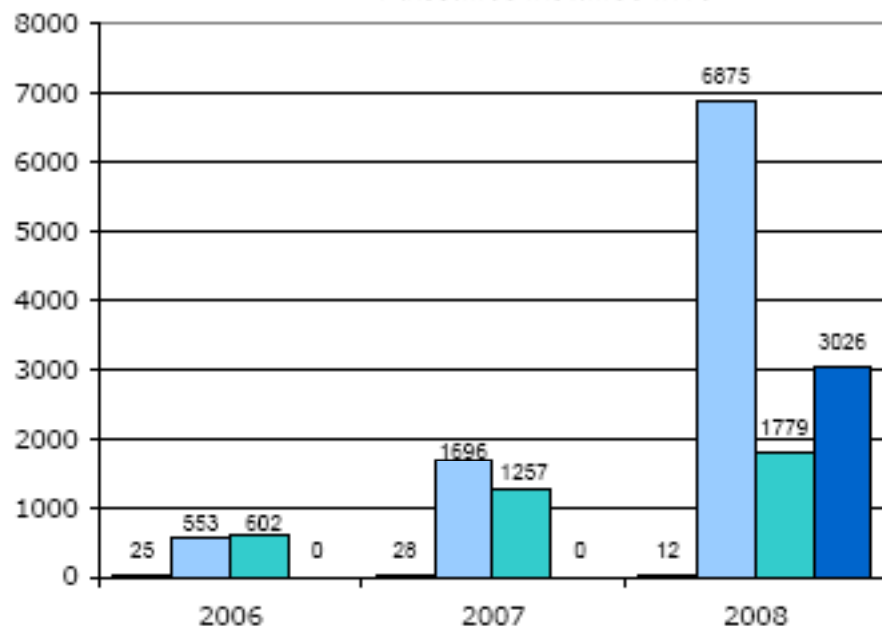
Evolutions des installations photovoltaïques Puissance installée kWc
